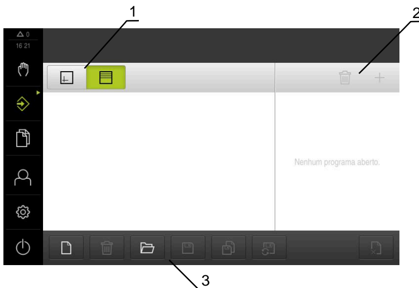
Figura 8: Menu Programação
